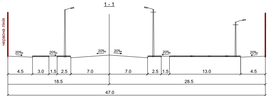
Поперечні профілі
